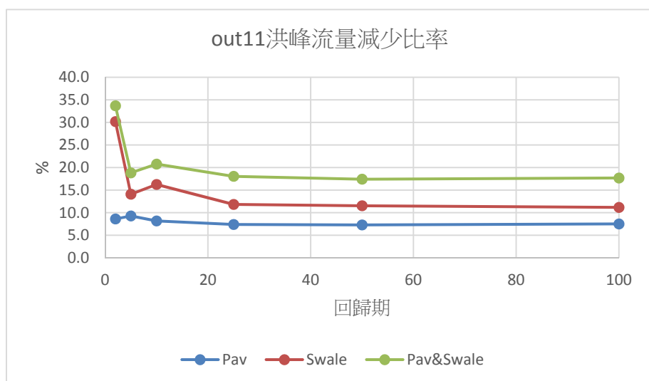
圖 31 不同回歸期下(1 小時延時)洪峰流量減少比率
