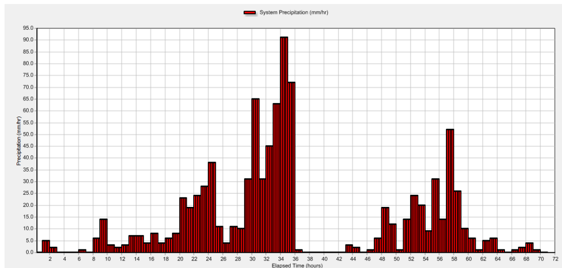
圖 24 納莉颱風時雨量歷線
