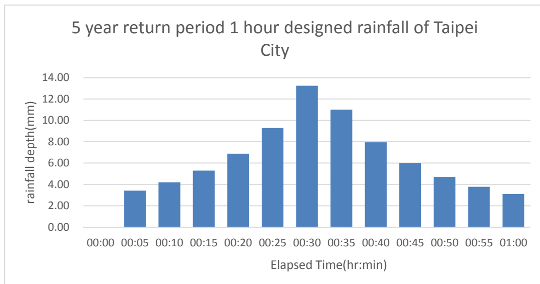
圖 18 一小時暴雨 5 年重現期降雨組體圖
