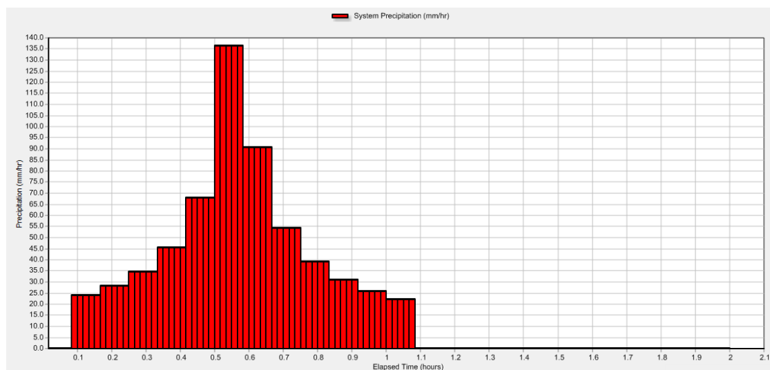
圖 20 降雨組體圖(兩年回歸期、降雨延時一小時)
