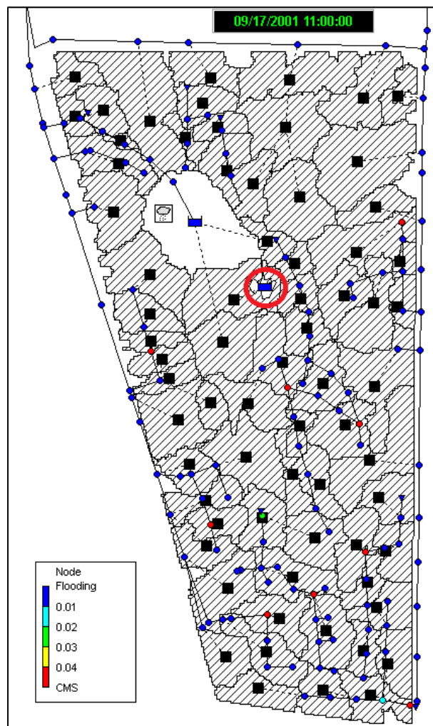
圖 32 新設生態池對排水影響(納莉颱風降雨歷線)
