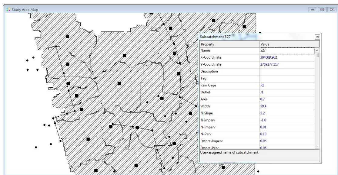
圖 16 SWMM 模式修改管線與陰井參數
