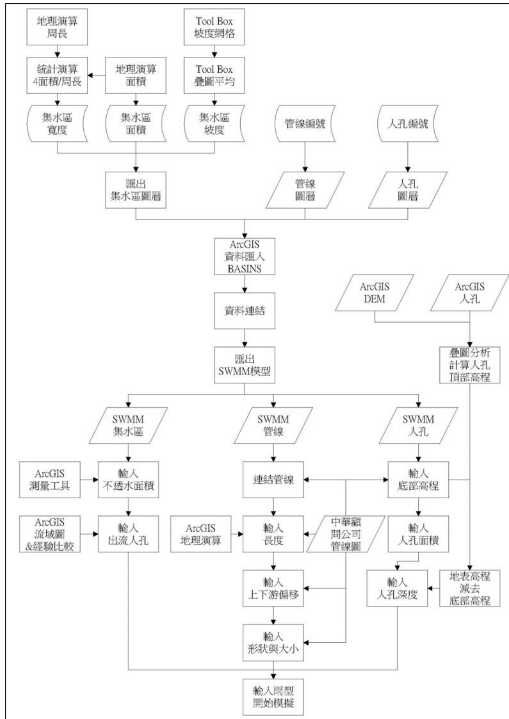
圖 17 排水模擬整體工作流程
