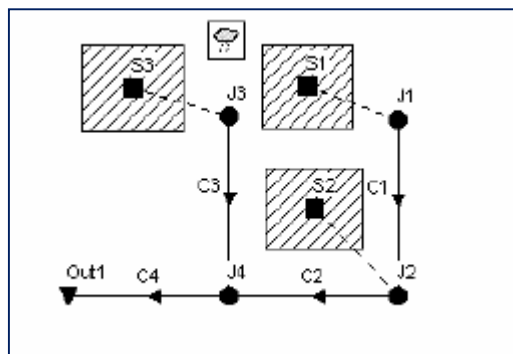
圖 5 排水系統地圖示意( 來源:SWMM 手冊)
