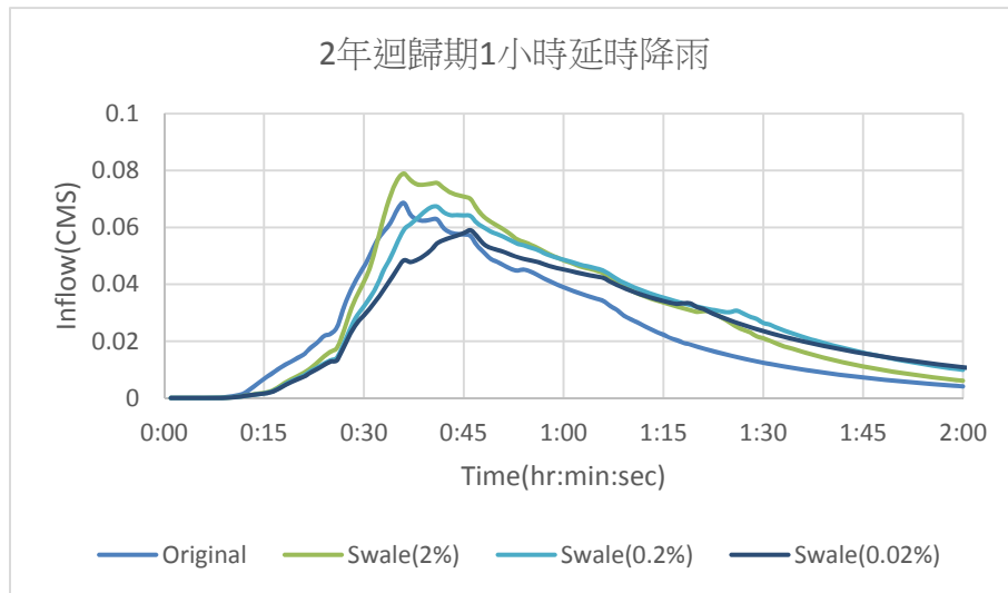
圖 28 不同坡度草溝(濕式溝)出流歷線比較
