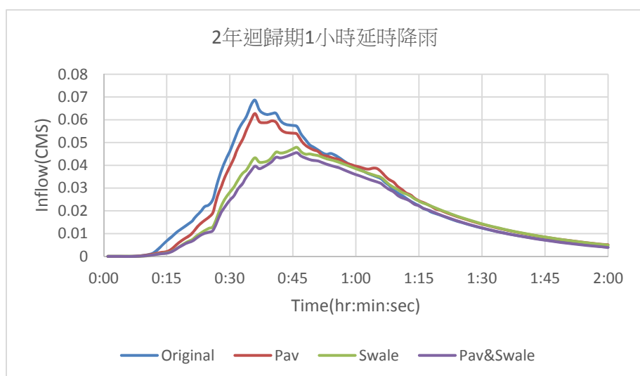
圖 30 設置不同 LID 之出流歷線比較
