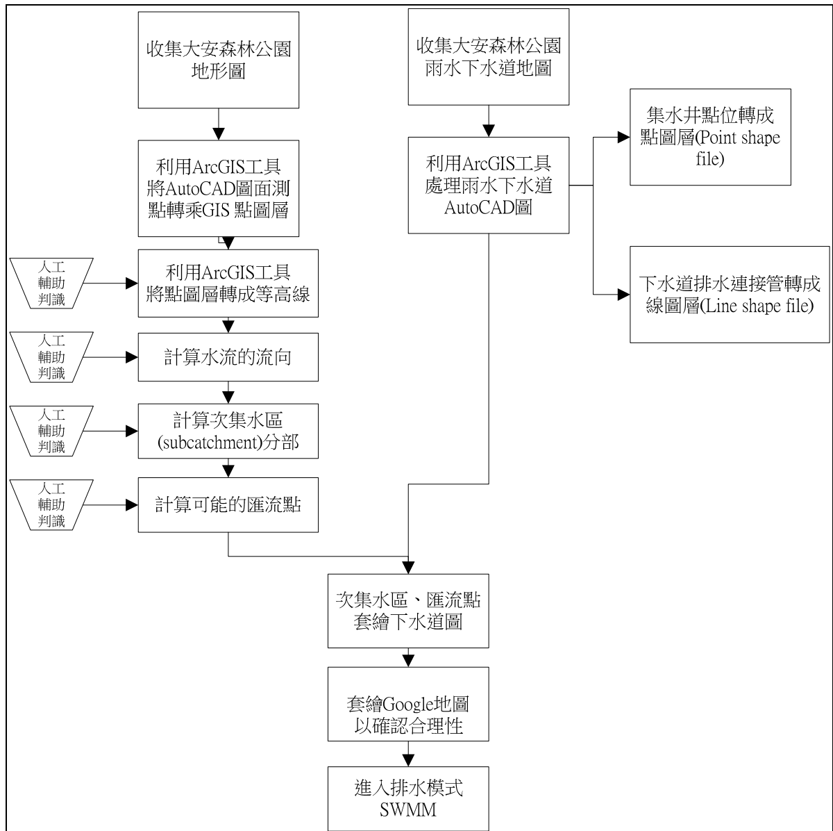
圖 6 大安森林公園劃分集水面積(catchment area)工作流程
