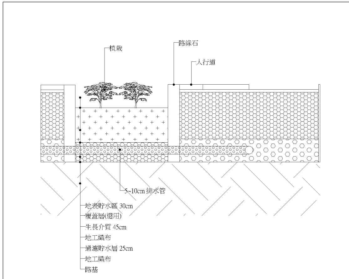
圖 27 草溝(乾式溝)配置圖(相當於線性雨水花園)
