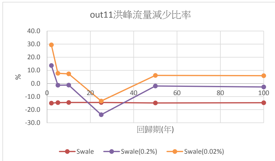
圖 29 不同回歸期下(1 小時延時)洪峰流量減少比率
