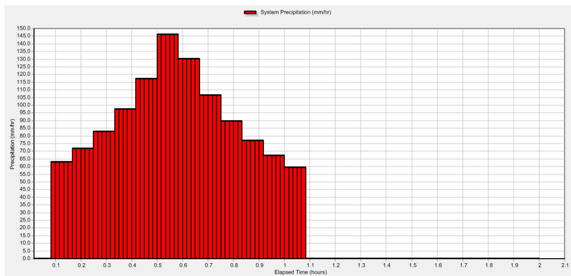
圖 22 降雨組體圖(25 年回歸期、降雨延時一小時)
