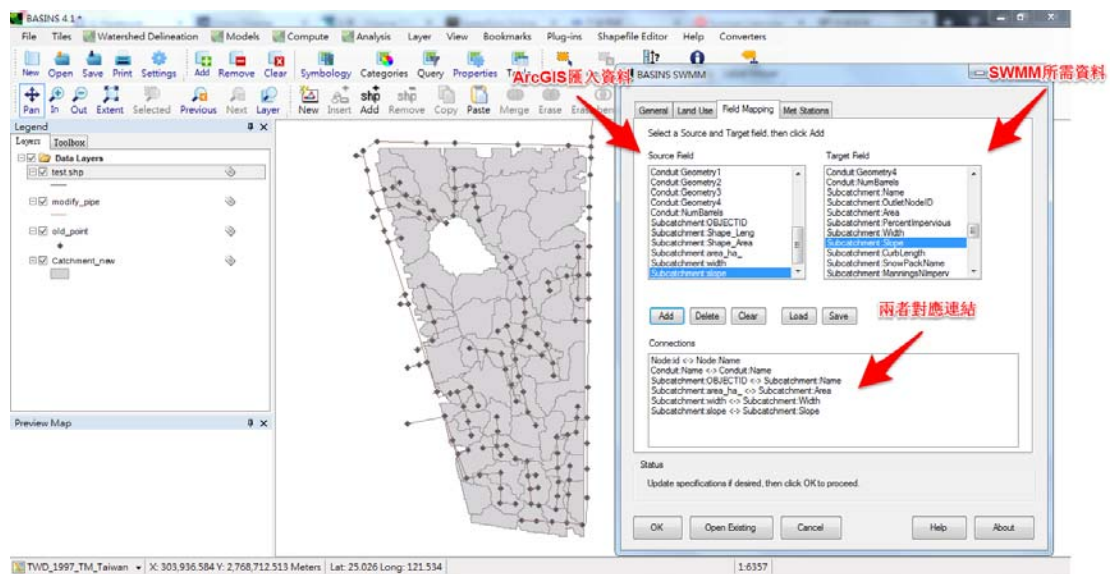
圖 15 利用 BASINS 軟體將 ArcGIS 轉 SWMM 相容格式
