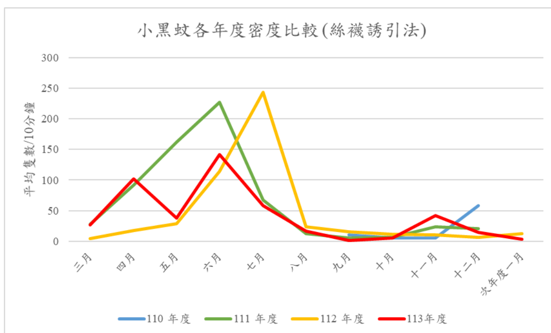
圖十七 小黑蚊各年度密度比較。110 年時小黑蚊的密度在 12 月後逐漸增加 111 年自三月起密度持續上升，在六月達到高峰，在 11 月後僅有些微上升。112 年度則是自五月起密度開始上升，在七月到達密度高峰，於八月後密度驟降。113 年度小黑蚊密度高峰位於四月、六月和十一月，主要是春末夏初為密度高峰。
