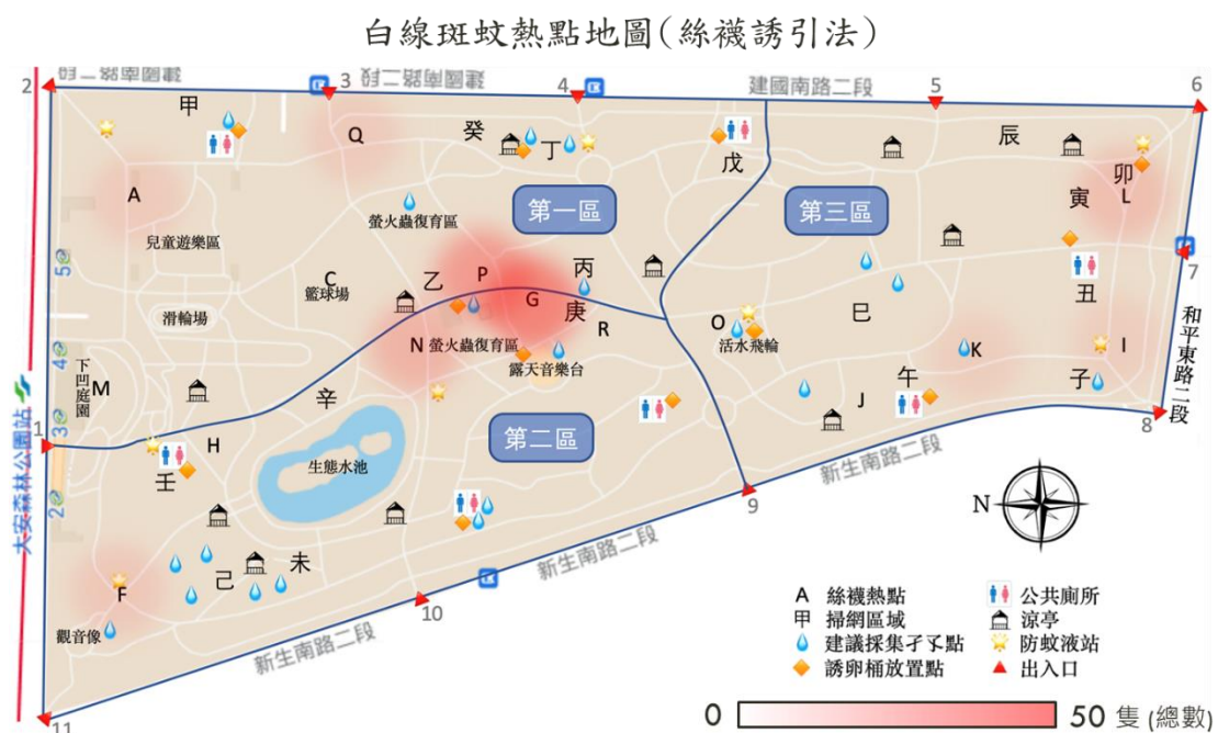
圖十四 113 年度白線斑蚊熱區圖。白線斑蚊在 G 區有顯著的族群數量，並以第二區的密度最高。
