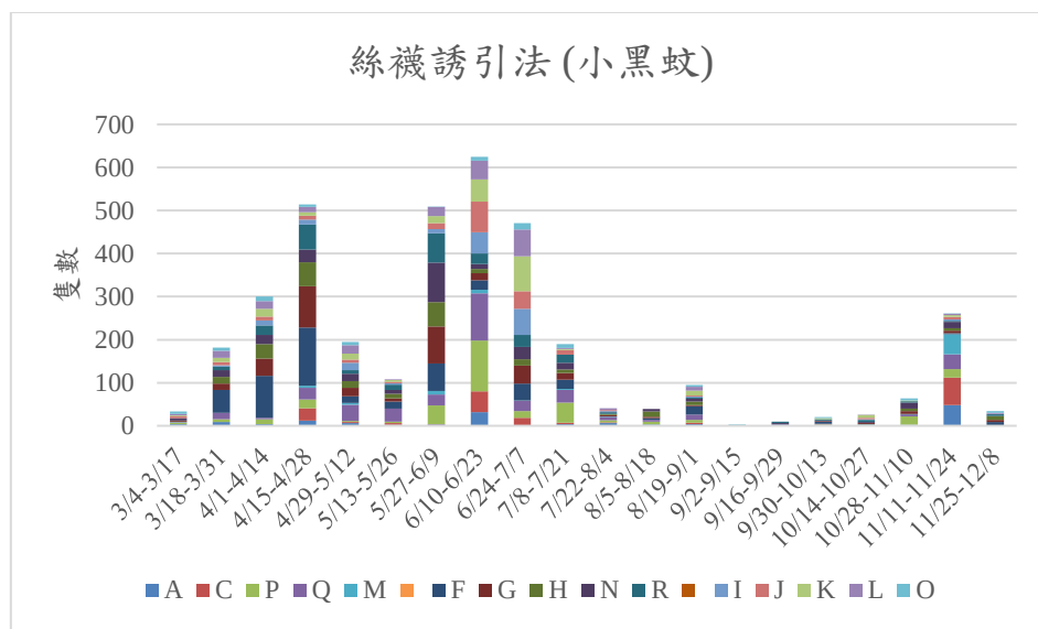
圖十九 113 年度絲襪誘引法小黑蚊各樣點密度，Y 軸為上午和下午四個監測時段絲襪誘引之小黑蚊總數量。
