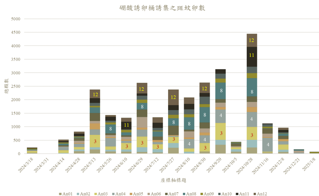
圖三十 113 年全年各時段誘卵桶監測之累積斑蚊卵數，白線斑蚊密度從五月開始上升，十月底有密度高峰，且 3、4、8、11 和 12 號樣點為熱點。
