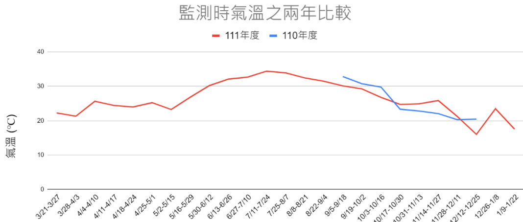
圖二十七 監測時氣溫之兩年比較。在10月中到12月初時，111年的氣溫比110年同時段來的高。
