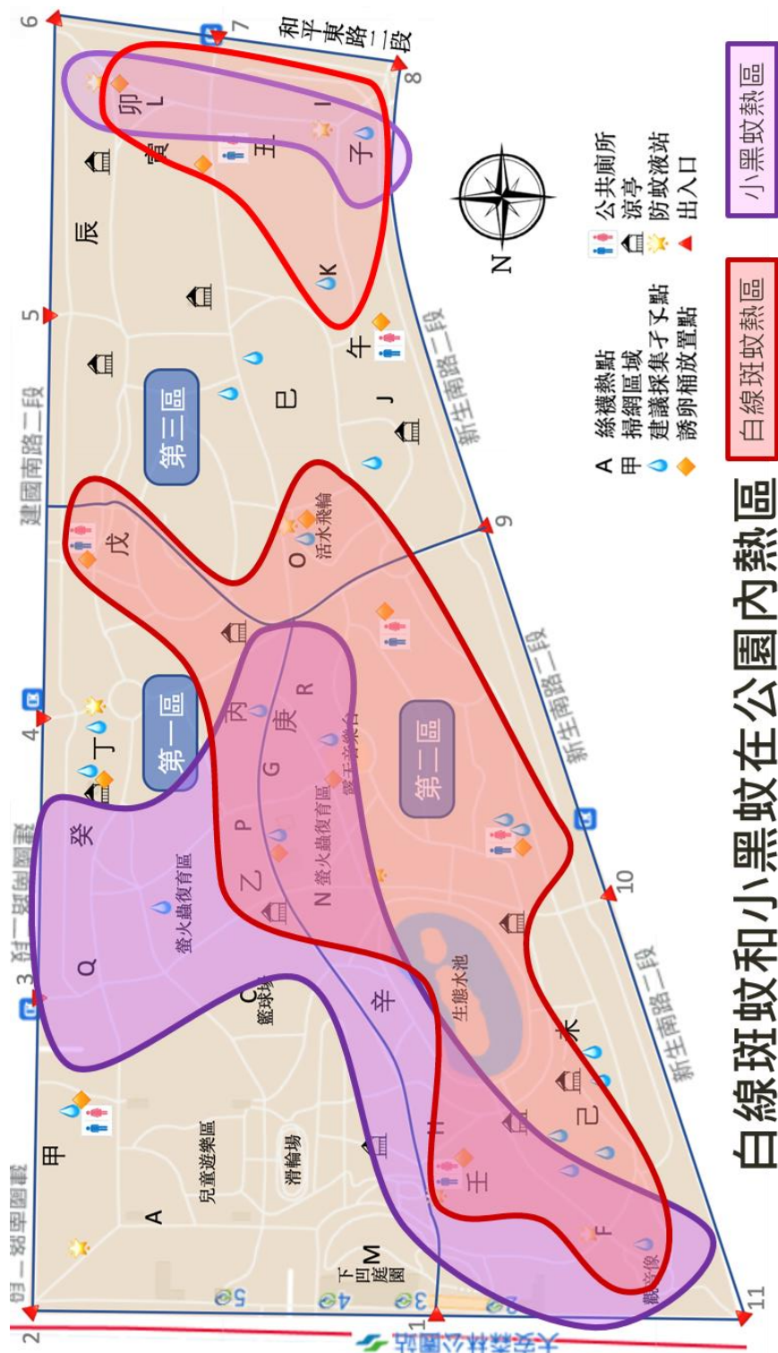
圖三十八 113 年度大安森林公園之小黑蚊及白線斑蚊熱點地圖。綜合成蟲掃網法、絲襪熱點法及硼酸溶液誘卵滅子桶監測之結果繪製，紫色區域範圍內為小黑蚊熱點，紅色區域範圍內為白線斑蚊熱點。
